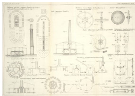
Abb. Schema Hoffmann Ringofen
